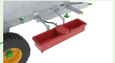
70 l Tränke mit Schwimmventil 1" (mit Verschlussventil für Transport), hinten oder seitlich angebracht.
